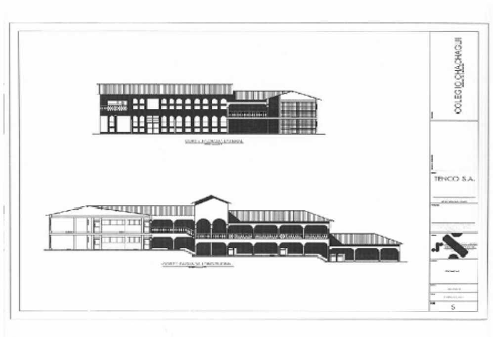
PLAN DE LA NOUVELLE ECOLE PRÉSCOLAIRE POUR LES ENFANTS DE SOL Y LUNA COLOMBIA
